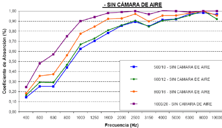
COEFICIENTE DE ABSORCIÓN ACÚSTICA EN CÁMARA REVERBERANTE (V=6.5m 3 )
