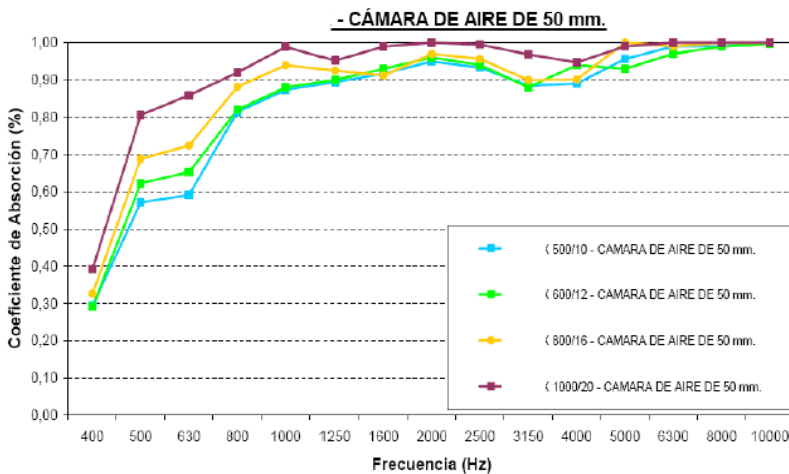
COEFICIENTE DE ABSORCIÓN ACÚSTICA EN CÁMARA REVERBERANTE (V=6.5m 3 )
